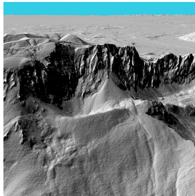
Bild 2: Digitales Geländemodell - 3D-Ansicht - Höllgrube an der Südseite der Benediktenwand
