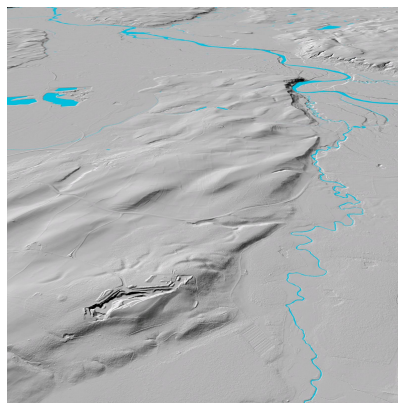
Bild 4: Digitales Geländemodell (3D-Ansicht) des Königsdorfer Drumlinfeldes
