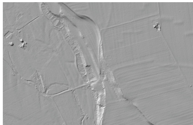
Bild 4: Terrassen im Digitalen Geländemodell
