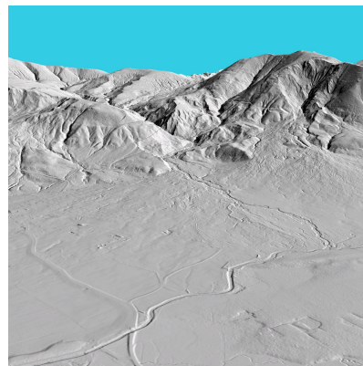
Bild 4: Digitales Geländemodell in 3D-Ansicht: Mündung des Lahngrabens und Mur-Schwemmkegel von Grafenaschau.
