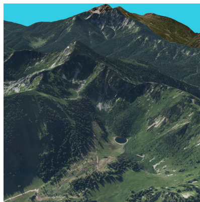
Bild 4: Oberes und unteres Kar unter dem Röthenstein in 3D-Ansicht (Geobasisdaten: (c) Bayerische Vermessungsverwaltung)
