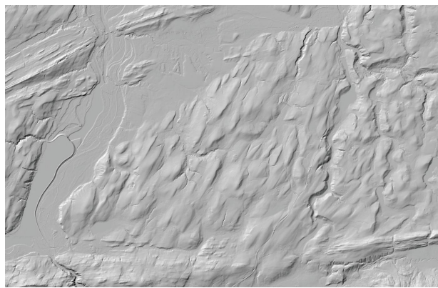
Bild 4: Drumlinfeld im Digitalen Geländemodell
