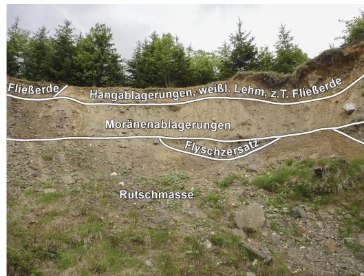
Bild 2: Interpretationen des Aufschlusses am Abriss im Schönleitenwald
