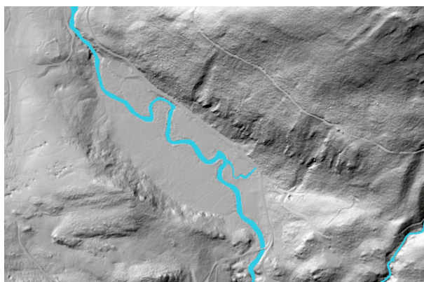
Bild 4: Digitales Geländemodell: Mäander der Valepp
