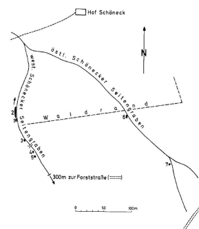
Abb. 11. Lageskizze des oligozänen Fischschiefers im westlichen Schöneck-Seitengraben. 1 = Fischschiefer, 2 = Stockletten, 3 = grauer, unregelmäßig vertikalender Mergel mit Stockletten, 4 = zone im bräunlichen Mergel, 5 = dunkelgrauer, verwitterter Mergel mit planktonischen Sandsteinlagen, 6 = dunkelgrauer, verwitterter Mergelschiefer mit rötlicher Einschiebung, 7 = schwarzer Mergel. Die Aufschlüsse 4-7 gehören der Buntmergel-Serie an.
