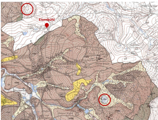
Bild 1: Lage des Maars Mytina (oben links), des Schlackenkegels Eisenbühl und des Maars Neualbenreuth (rechts unten) in der Geologischen Karte 1:15.000
