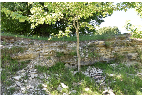
Bild 3: Aufschluss von gebankten Kalk- und Mergelsteinen
