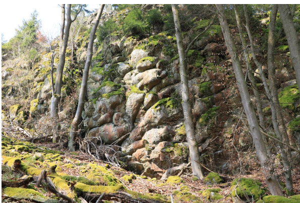
Bild 3: Kissenförmig abgesonderter Diabas ("Pillows")
