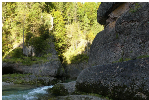
Bild 4: Engstelle der Scheibum: Konglomerate der Weißbach-Schichten
